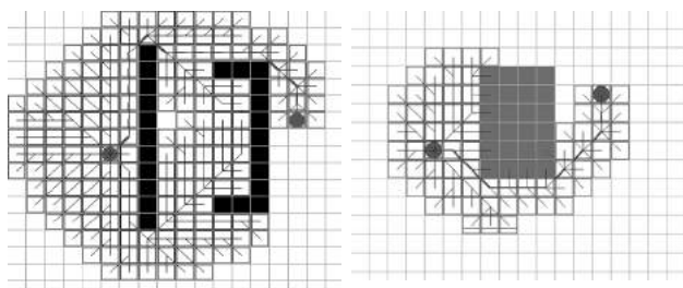
Рис.1. Примеры работы Алгоритма A*.
