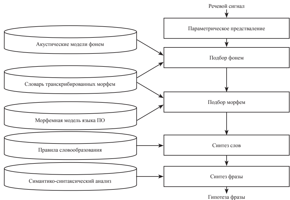
Рис. 1. Система интегрального распознавания и понимания речи SIRIUS
