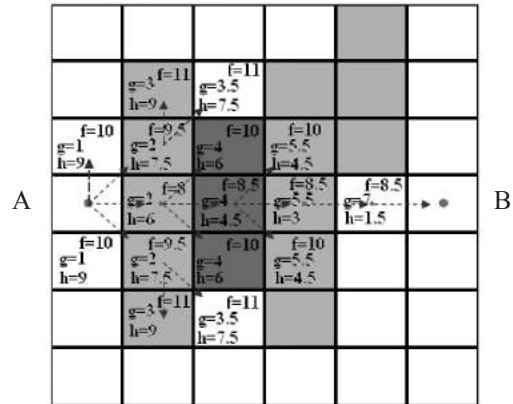
Рис. 3. Пример решения задачи нахождения оптимального пути с помощью алгоритма A*
