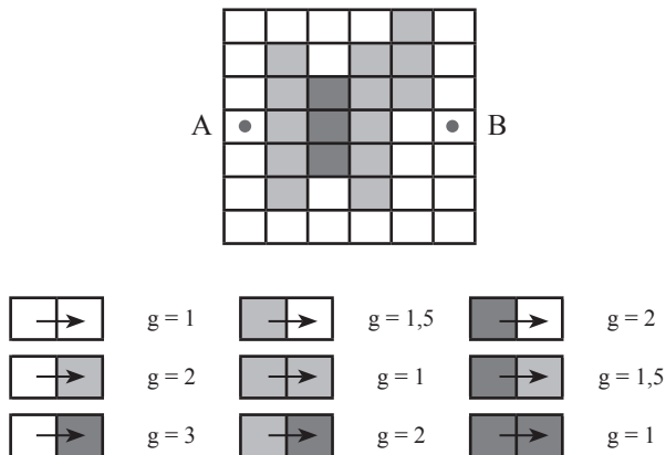
Рис. 2. Растровая модель рельефа со стоимостью перехода между местностями различных типов
