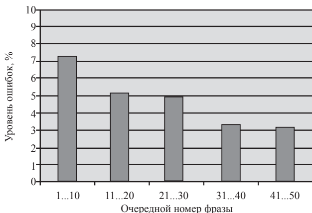
Рис. 3. Уровень ошибок распознавания в зависимости от номера фразы диктора
